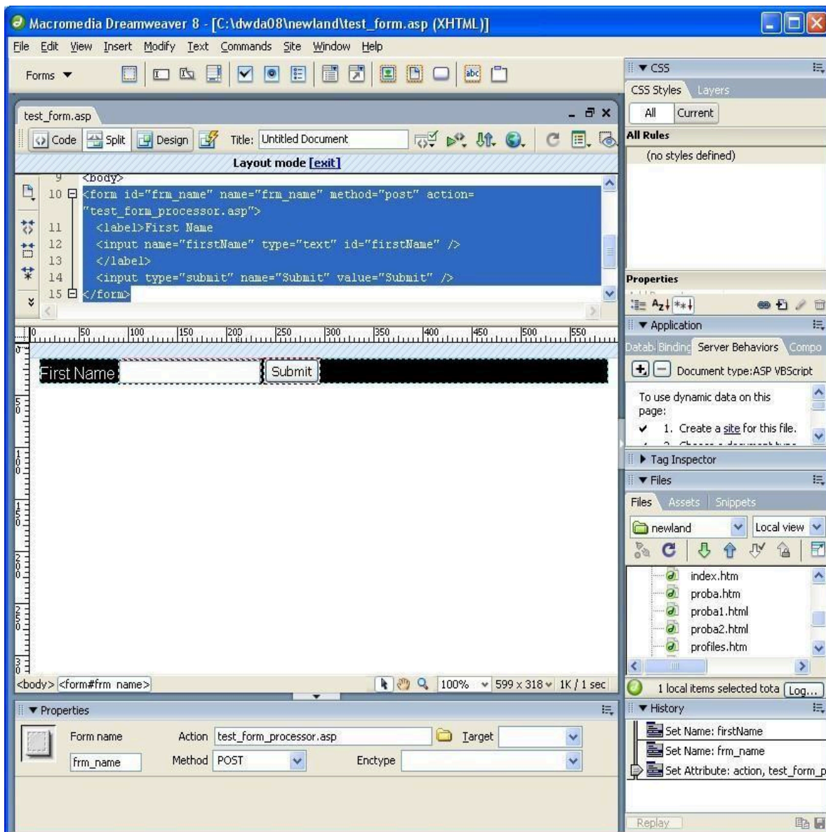
Рис. 3. Выделение формы с помощью селектора тегов
